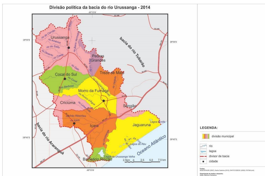
Figura 1: Mapa da bacia do rio Urussanga.
