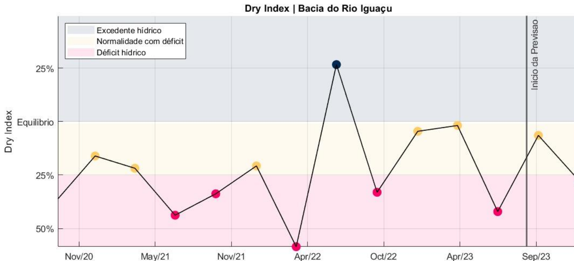
Figura 6. IH para a Bacia do Rio Iguaçu. Fonte: SPEHC ( Rodada de Setembro/2023 ).
