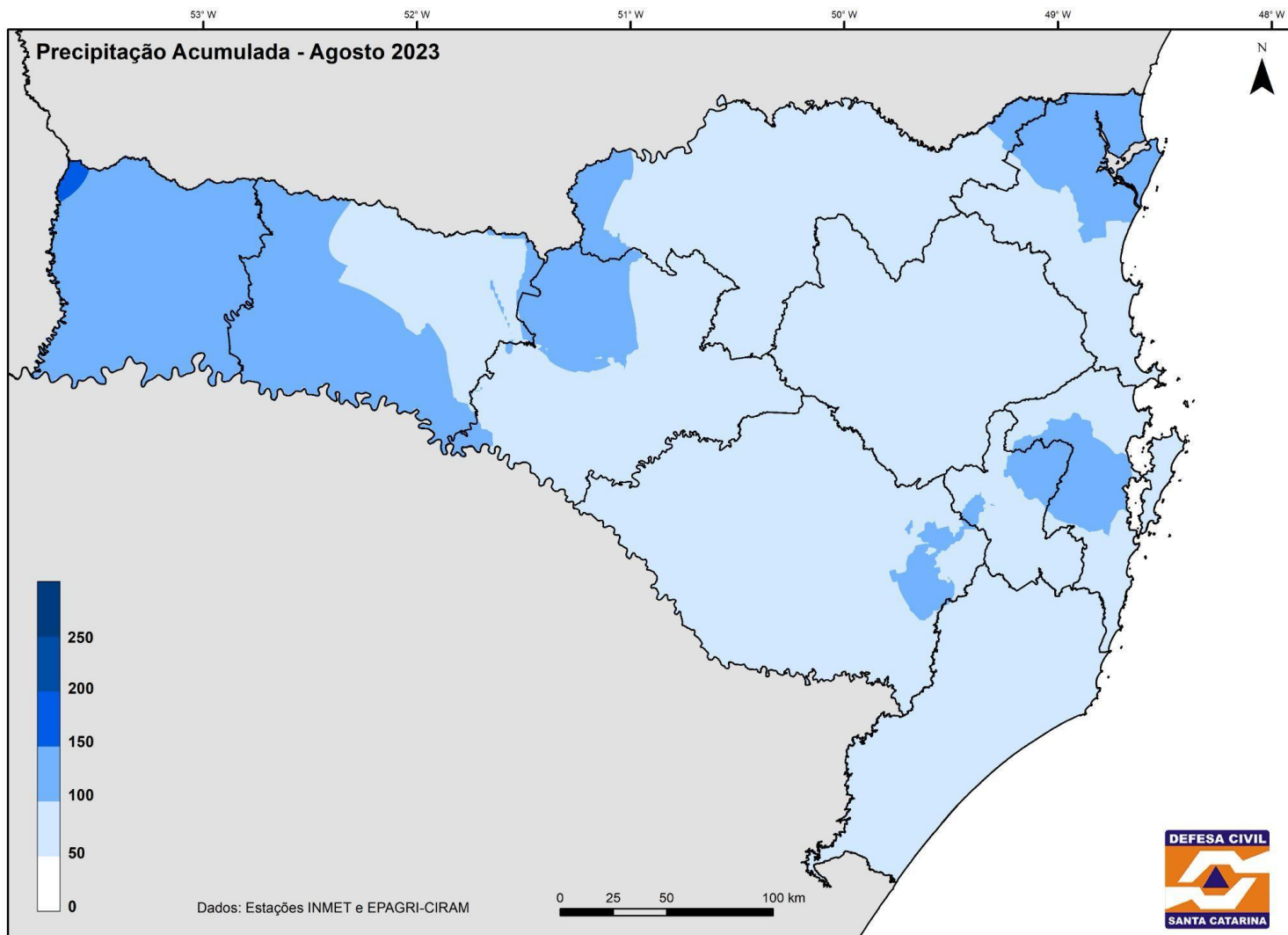
Figura 1. Distribuição espacial da chuva acumulada em agosto de 2023, em Santa Catarina.
