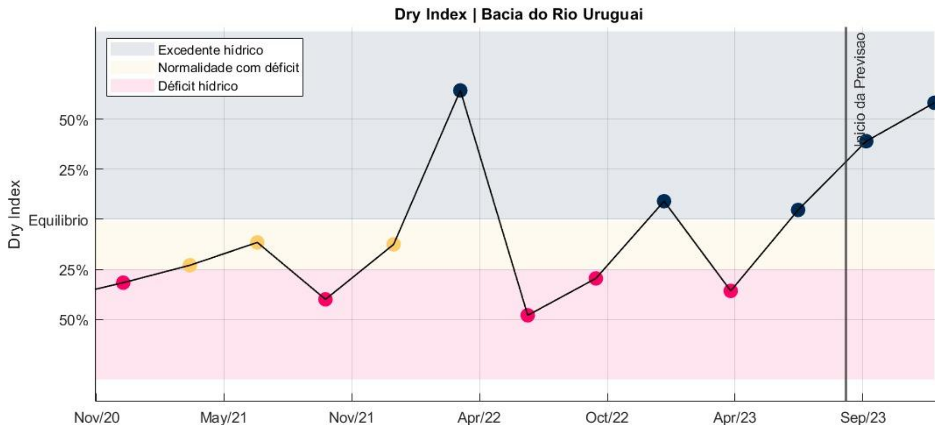
Figura 7. IH para a Bacia do Rio Uruguai. Fonte: SPEHC ( Rodada de Setembro/2023 ).
