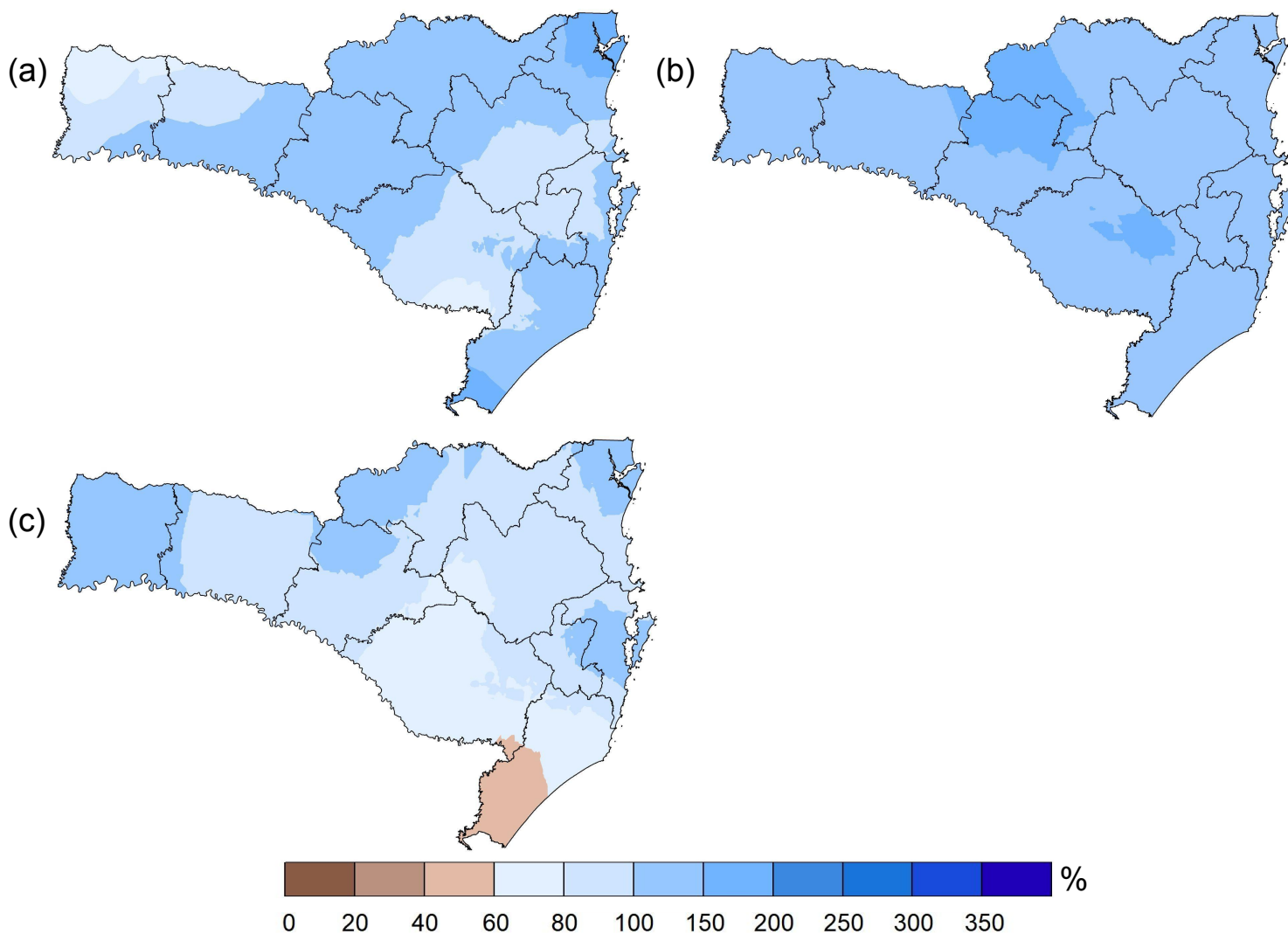
Figura 3. Distribuição espacial da porcentagem de chuva, em relação à média mensal, no mês de: (a) junho, (b) julho e (c) agosto. Dados: Epagri/Ciram, ANA e INMET. Arte: Defesa Civil de Santa Catarina.
