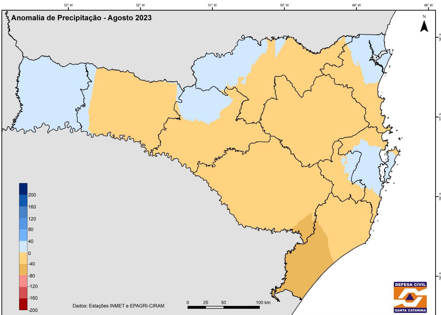
Figura 2. Distribuição espacial da anomalia de chuva em agosto de 2023, em Santa Catarina. Dados: Epagri/Ciram, ANA e INMET. Arte: Defesa Civil de Santa Catarina.
