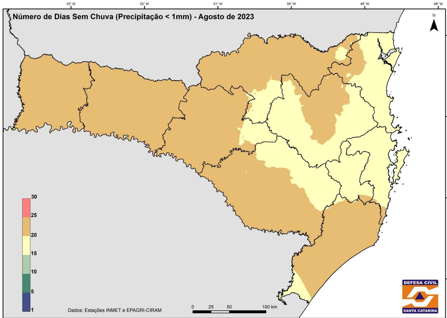
Figura 4. Distribuição espacial do número de dias sem chuva no mês de agosto de 2023.
