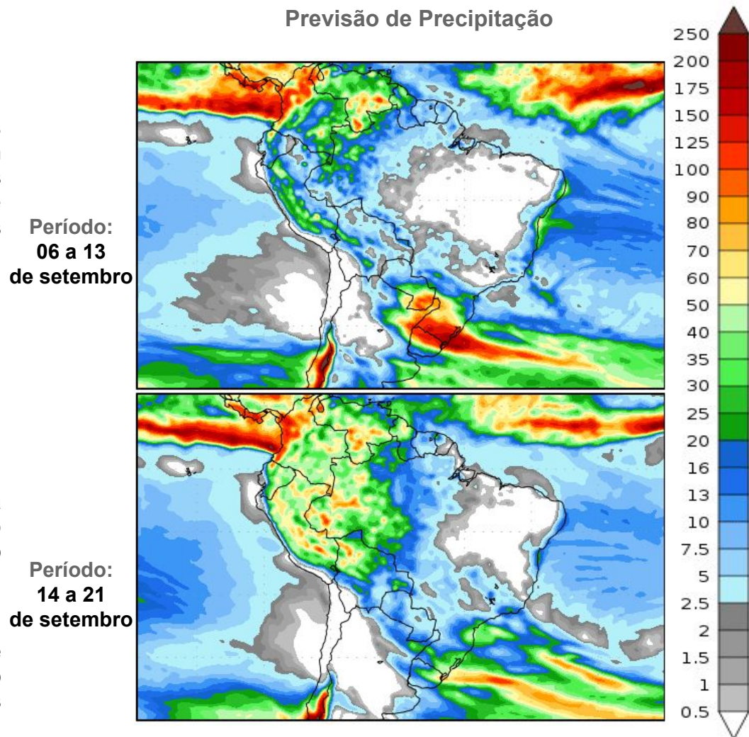
Figura 5. Acumulados de precipitação previstos entre os dias 06 e 13 (imagem superior) e 14 e 21 de setembro de 2023 (imagem inferior), segundo o modelo GFS. Fonte: COLA (Center for Ocean-Land-Atmosphere-Studies).
