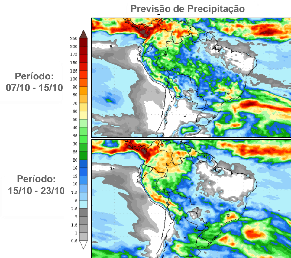
Figura 5. Acumulados de precipitação previstos para o decorrer do mês de outubro; entre os dias 07 e 15 (imagem superior) e 15 a 23 (imagem inferior), segundo o modelo GFS.
