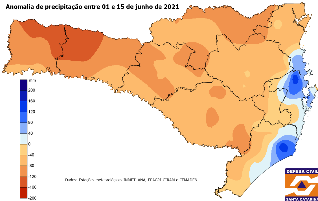
Figura 2. Distribuição espacial da anomalia de chuva na primeira quinzena de junho de 2021, em Santa Catarina. Dados: Epagri/Ciram, ANA e INMET. Arte: Defesa Civil de Santa Catarina.
