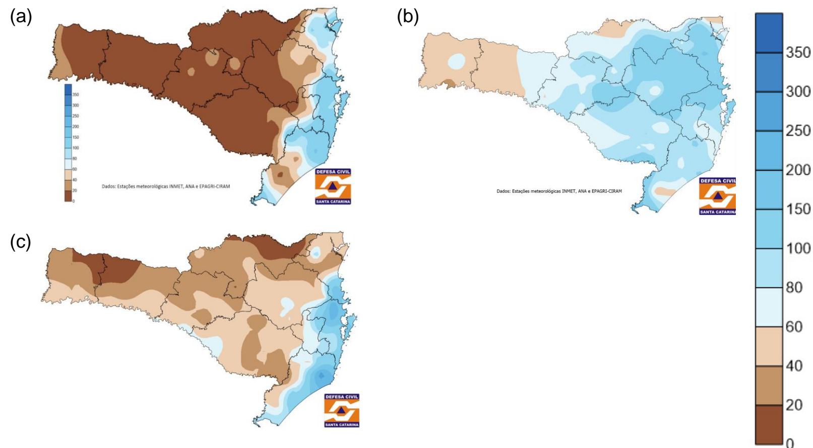
Figura 4. Distribuição espacial da porcentagem de chuva, em relação à média mensal, no mês de: (a) abril (b) maio e (c) primeira quinzena de junho de 2021. Dados: Epagri/Ciram, ANA e INMET. Arte: Defesa Civil de Santa Catarina.
