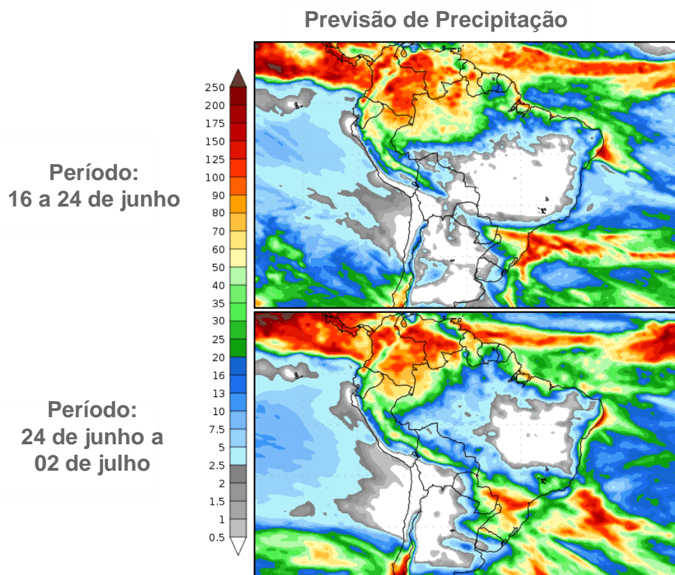
Figura 5. Acumulados de precipitação previstos entre os dias 16 e 24 de junho (imagem superior) e 24 de junho a 02 de julho de 2021 (imagem inferior), segundo o modelo GFS. Fonte: COLA ( Center for Ocean-Land-Atmosphere-Studies ).
