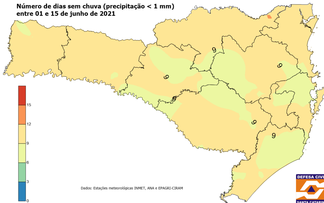
Figura 3. Distribuição espacial do número de dias sem chuva na primeira quinzena de junho de 2021. Dados: Epagri/Ciram, ANA e INMET. Arte: Defesa Civil de Santa Catarina.
