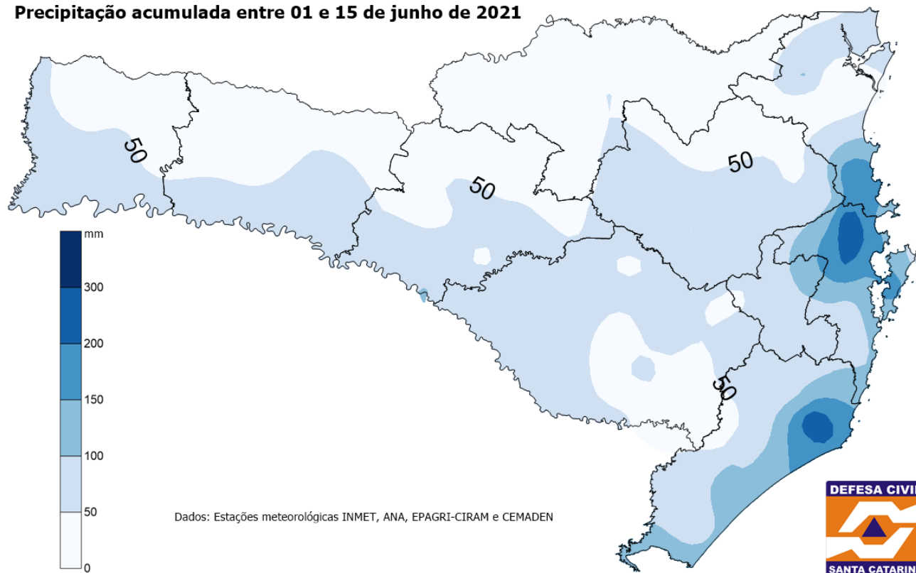
Figura 1. Distribuição espacial da chuva acumulada na primeira quinzena de junho de 2021, em Santa Catarina. Dados: Epagri/Ciram, ANA e INMET. Arte: Defesa Civil de Santa Catarina.
