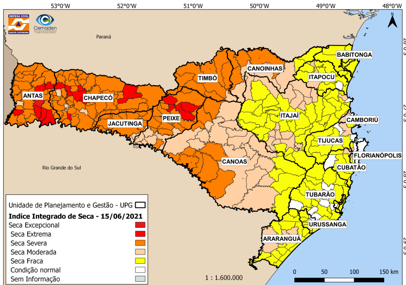
Figura 8. Classificação do IIS associado por município/região hidrográfica, referente a data de 15/06/2021. Fonte: Adaptado de CEMADEN/ANA.
